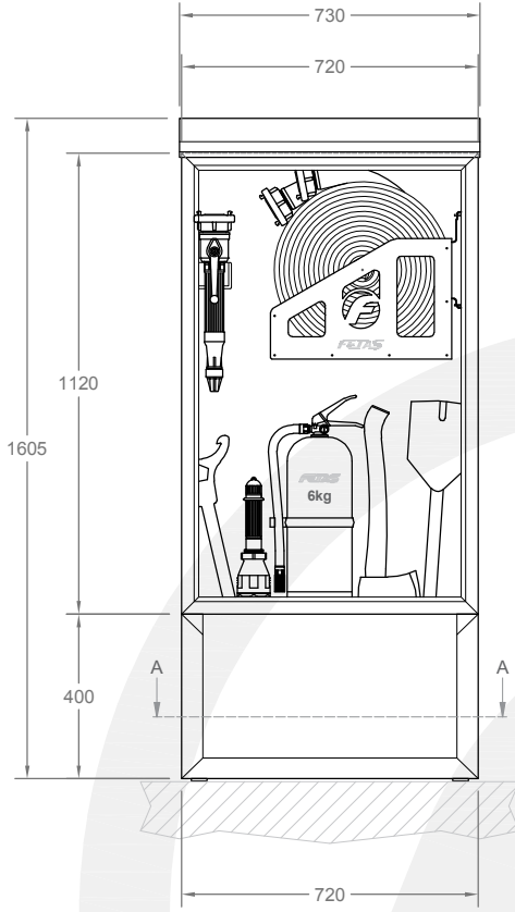
ÖN GÖRÜNÜŞ FRONT VIEW
