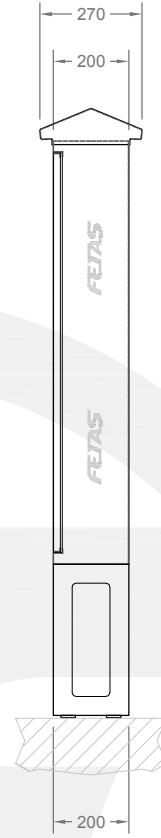
YAN GÖRÜNÜŞ SIDE VIEW
