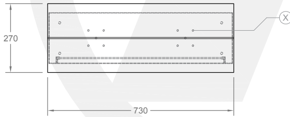
ÜST GÖRÜNÜŞ TOP VIEW
