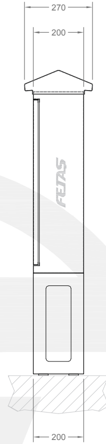
YAN GÖRÜNÜŞ SIDE VIEW
