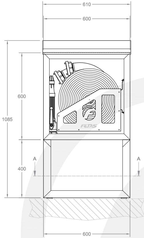
ÖN GÖRÜNÜŞ FRONT VIEW
