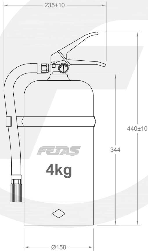
ÖN GÖRÜNÜŞ FRONT VIEW
