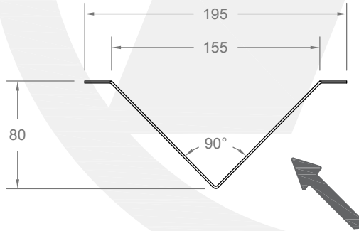
ÜST GÖRÜNÜŞ TOP VIEW
