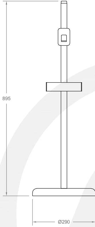
ÖN GÖRÜNÜŞ FRONT VIEW
